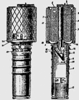
Устройство универсальной наступательно-оборонительной гранаты
