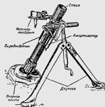
Миномет образца 1940 года
